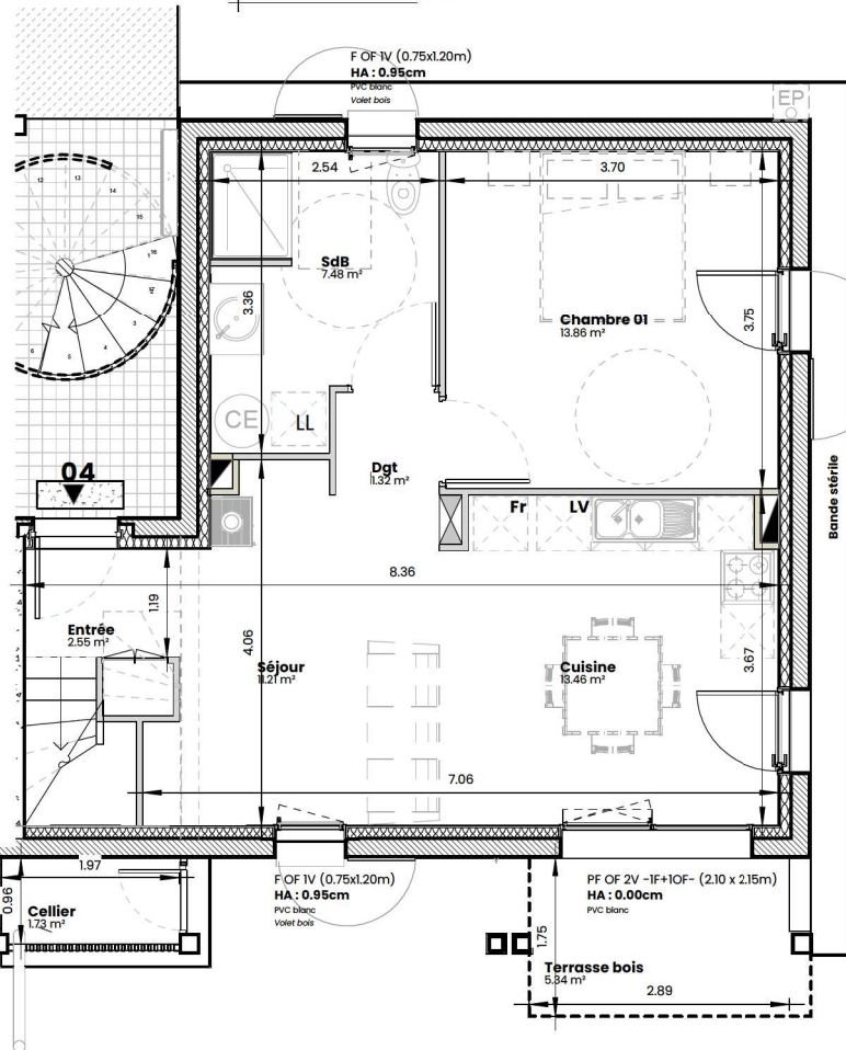
Plan RDC
