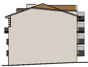
Façade Ouest
