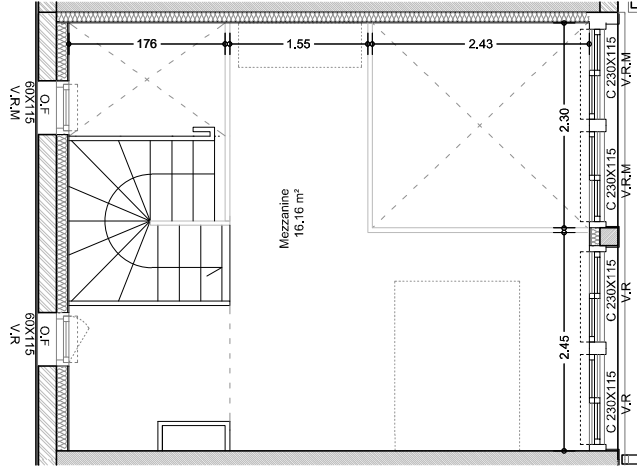
C03 _ Plan R+1/50
